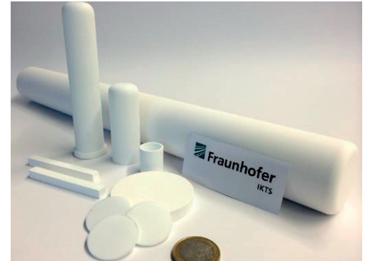
Abb. 3: Verschieden geformte Elektrolyte aus Na-β"-Aluminat.
