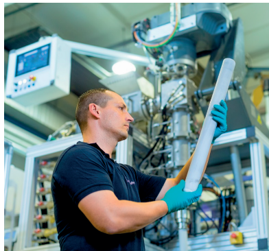
Abb. 2: Elektrolytrohr aus Na-β"-Aluminat vor der Sinterung.
