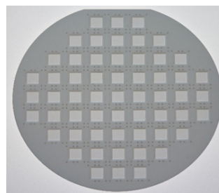
Bondbarer LTCC-Wafer mit eingefügten Kavitäten und Au-Vias zur ASIC-Integration.
