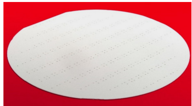
Polierter LTCC-Wafer mit Gold-Vias für das anodische Bonden mit Silizium-MEMS-Wafer.
