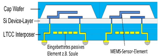
Prinzipskizze Wafer-Level-Packaging von LTCC-Keramik mit Si-MEMS-Wafer.
