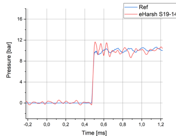
Kennlinien des Drucksensors unter dynamischer Druckänderung (Stoßrohrmessung).
