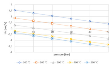
Kennlinien des Drucksensors im Temperaturbereich 100–500 °C.
