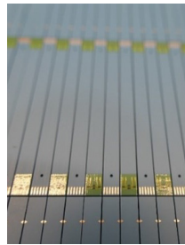
Mehrlagenkeramisches Sensorelement in Nutzenfertigung.
