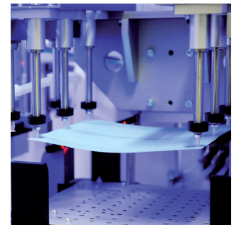
Mikrobearbeitungszentrum für keramische Multilayer.
