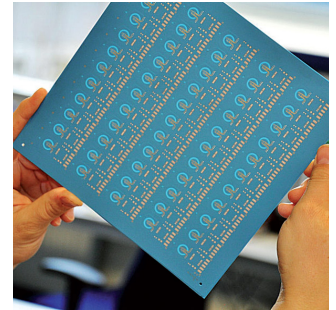
LTCC-basierte Drucksensoren (Nuten 8" x 8").
