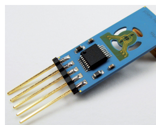
LTCC-basierter Drucksensor.
