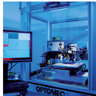
Abscheidung von Funktionsschichten mittels Aerosoldruck.
