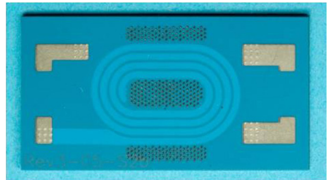
100 W-Hochstrom-Transformator in LTCC mit ferritischen Vias (Volumen = 0,8 cm 3 ).
