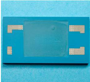
100 W-Hochstrom-Transformator in LTCC mit monolithisch integrierten Ferritplatten.
