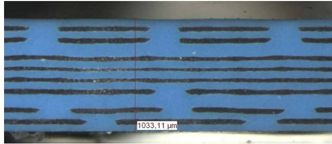
Schliff-Ansicht eines gesinterten LTCC-Transformators mit 50 µm Silberschichtdicke und 8 Metallisierungsebenen.
