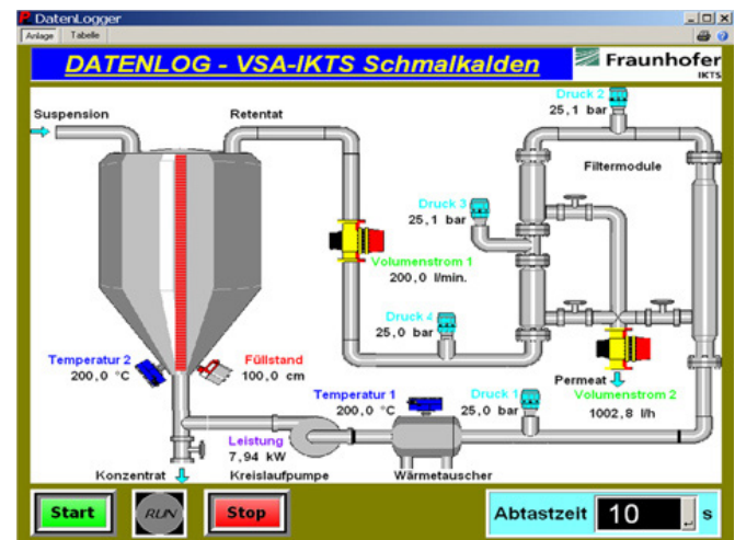
Flussbild der Filtrationsanlage.
